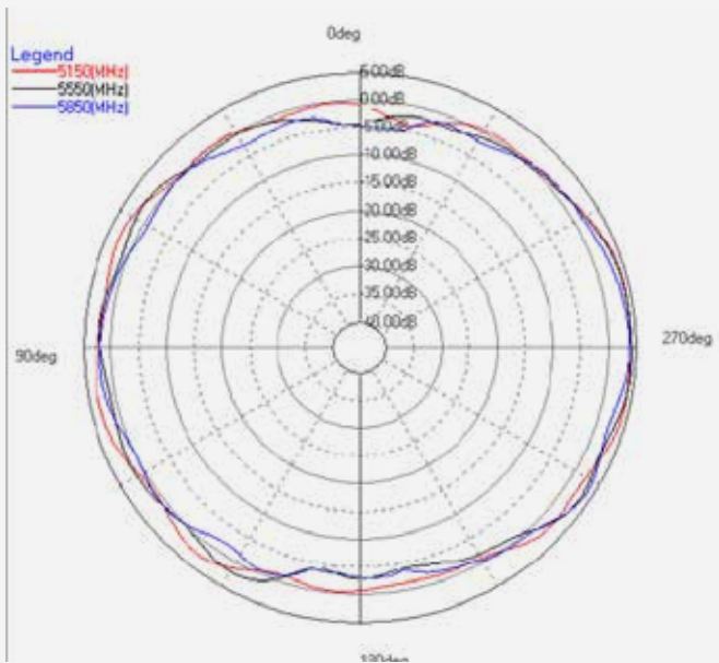
5G (PHI=0)
