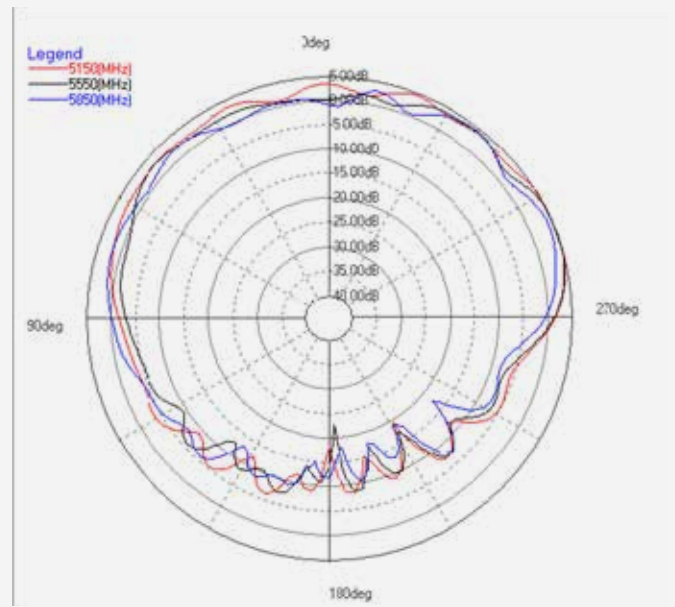
5G (PHI=90)
